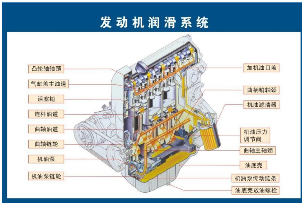
图9 发动机润滑系统
