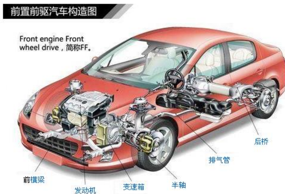
图2 发动机在汽车上的常见布置
