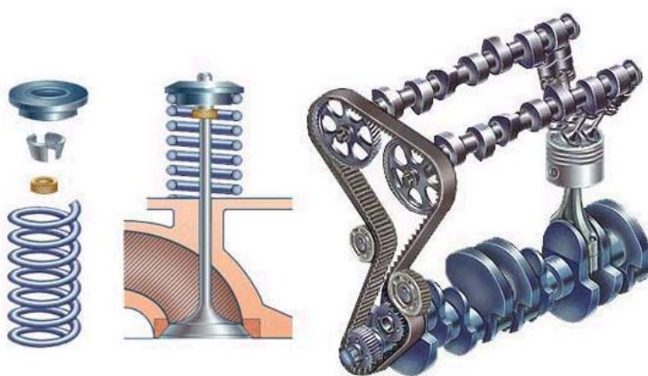
图5 配气机构
