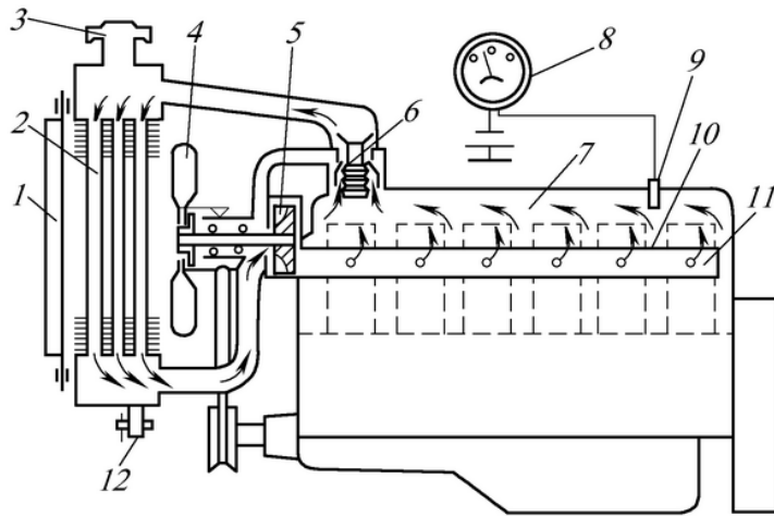
强制循环水冷系统
