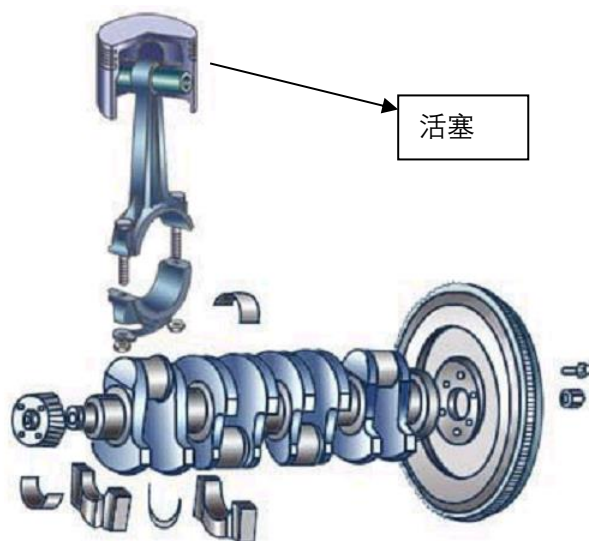
图4 曲柄连杆机构
