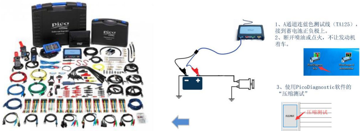
图13 发动机信号采集仪器
