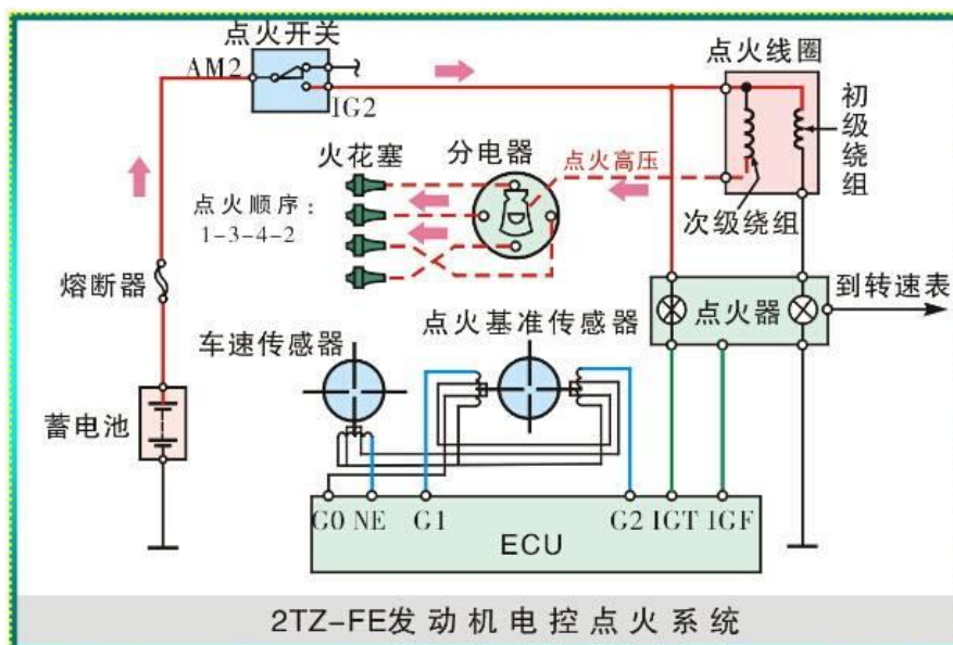
图7 发动机点火系统
