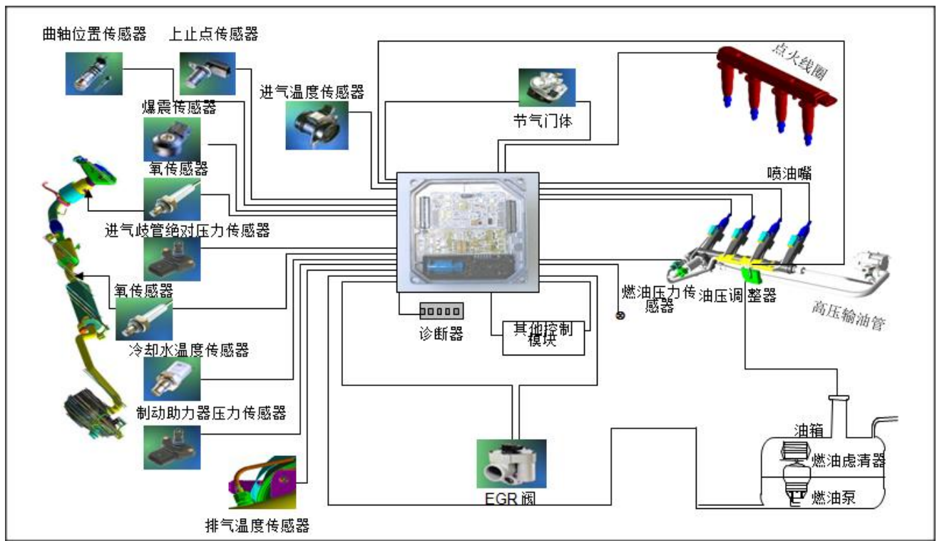
图6 电子控制供给系统
