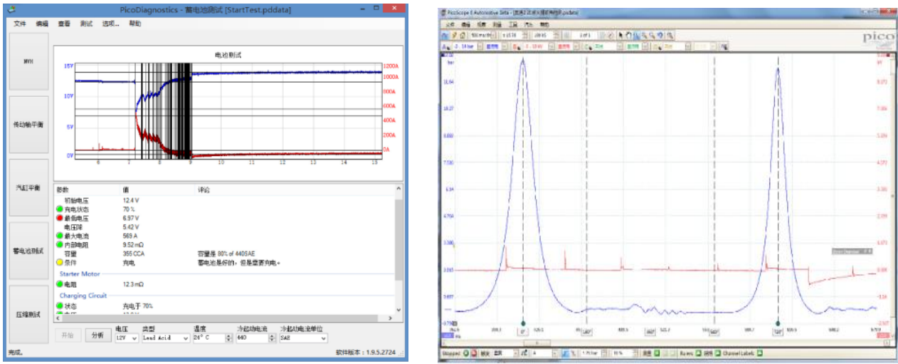
图14 发动机信号采集样例
