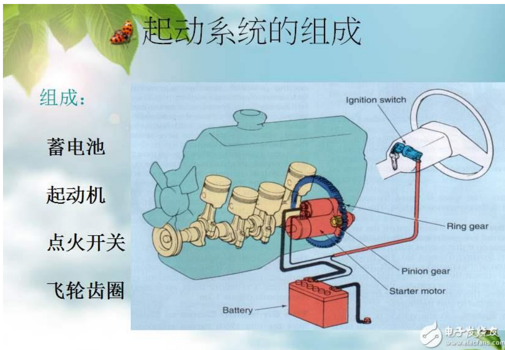
图10 发动机起动系统
